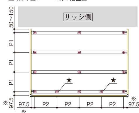
図2) 床下囲いベース材の配置図
