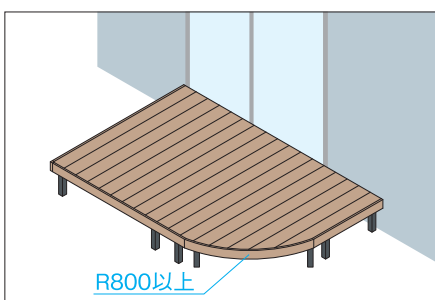
アール納まり
