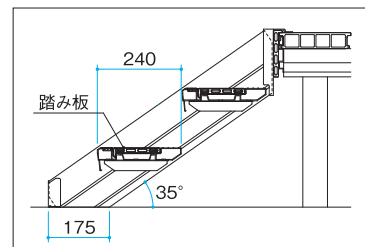
ロング(H=700用)
