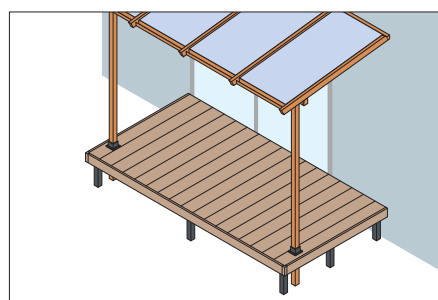
テラス柱納まり
