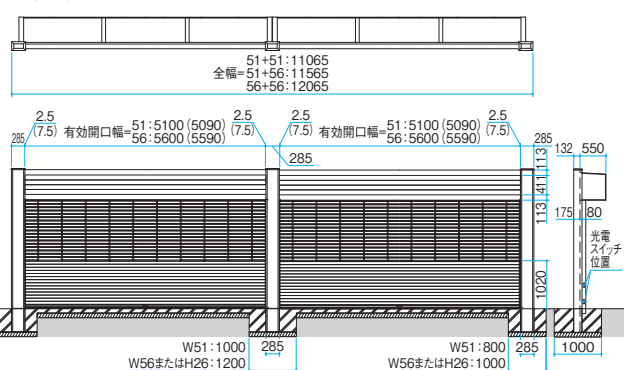
4台駐車用
