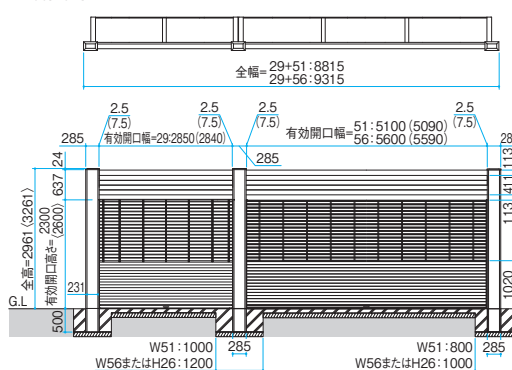
3台駐車用
