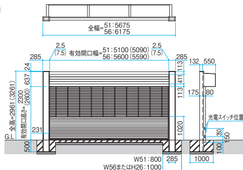
2台駐車用
