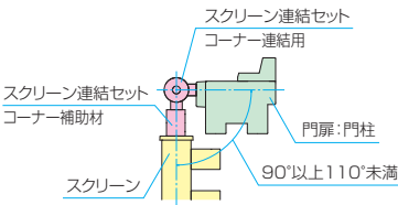
MFL-1・M1 門柱+門扉+ランマ 内開き施工 セット価格表(スクリーンH=2550mm・3000mm)の場合 3
