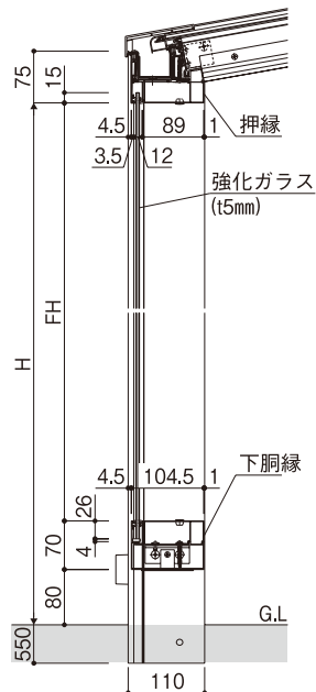
基本フレーム納まり
