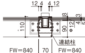
多連結フレーム納まり
