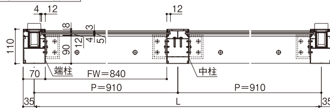
多連結フレーム納まり
