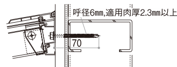
軽量鉄骨用部品
