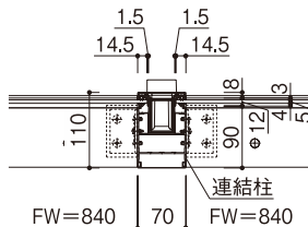
多連結フレーム納まり
