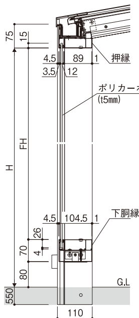
基本フレーム納まり
