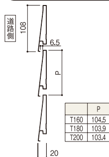
たて断面
