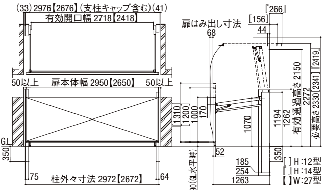
ハイルーフタイプ 図は30-10サイズ
