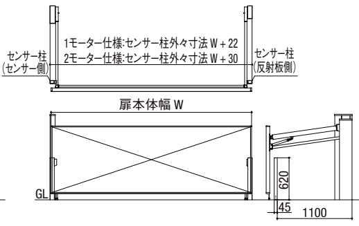
ハイルーフタイプ 図は30-10サイズ
