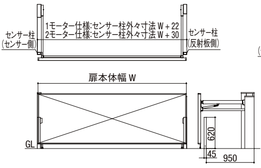
標準タイプ 図は30-10サイズ
