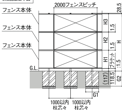
3段施工基本図
