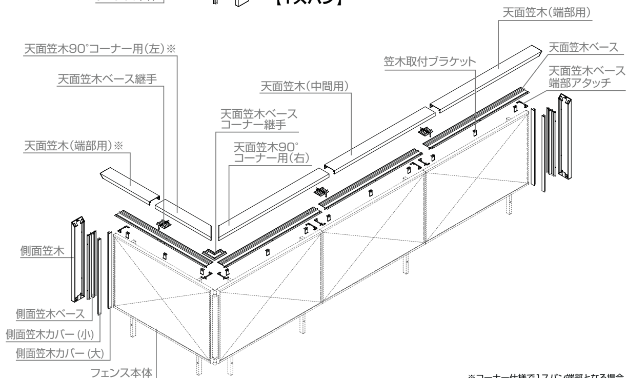
【コーナー(図は出隅)】
