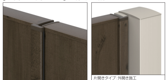
片開きタイプ：外開き施工
