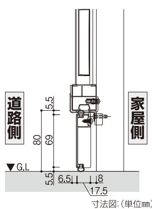
寸法図:(単位mm)
