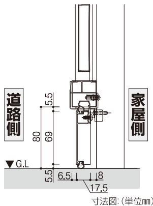
YS3FS型 T160
