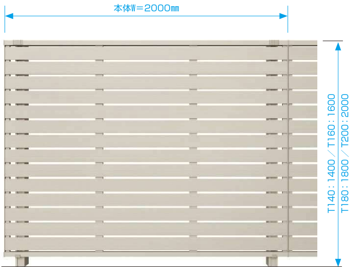
YS3S型 T160
