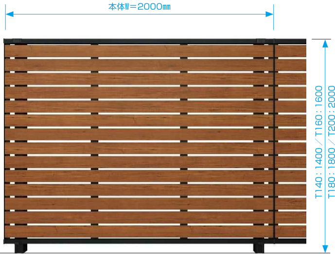
YS3FS型 T160
