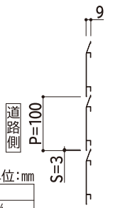
格子断面
