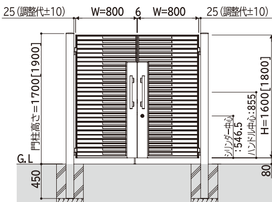
※本図は内開き右勝手（道路側） ※[ ]寸法は、H18の場合です。
