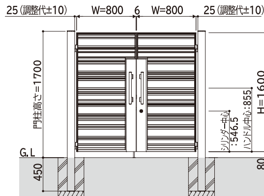
※本図は内開き右勝手（道路側）
