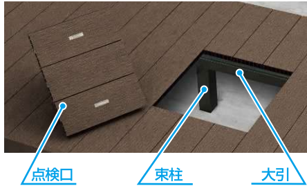
リウッドデッキ 200 EG (レッドブラウン色)
