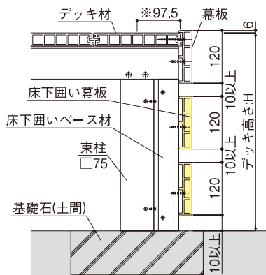
図1)床下囲い幕板配置図(2段取付け例)
