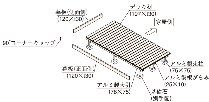
ナチュラルブラウン色 (Sタイプ 幅3651×奥行1820mm (2間×6尺) / 独立式 リウッド ステップ2型)
